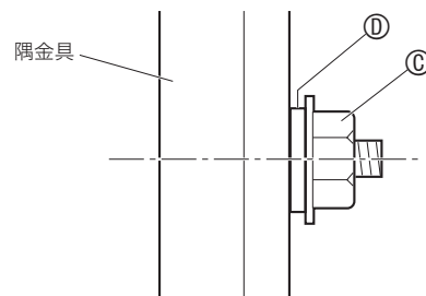
<正しい取り付け>
