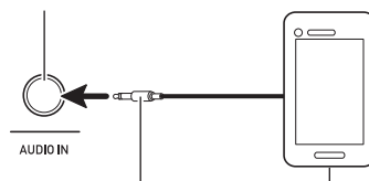
ステレオミニフォンプラグ(ミニTRSフォン) 携帯オーディオプレーヤーなど
