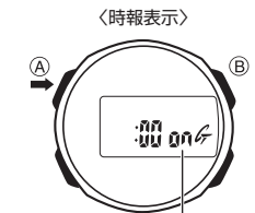
時報ONのときは "on" 表示 / 時報OFFのときは "oF" 表示
